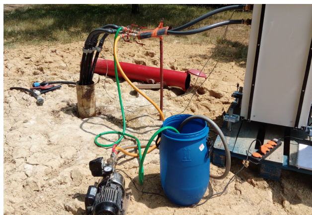
Test de réponse thermique sur la première sonde à l'école du bois d'amour - Saint Benoit (86)
