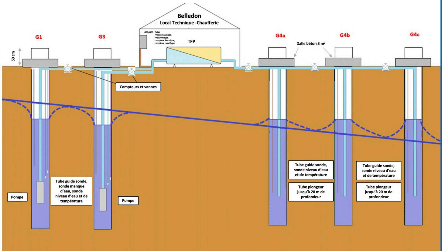
Dispositif Géothermie Belledone en boucle ouverte au Futuroscope pour le futur centre Aquascope et bâtiments
